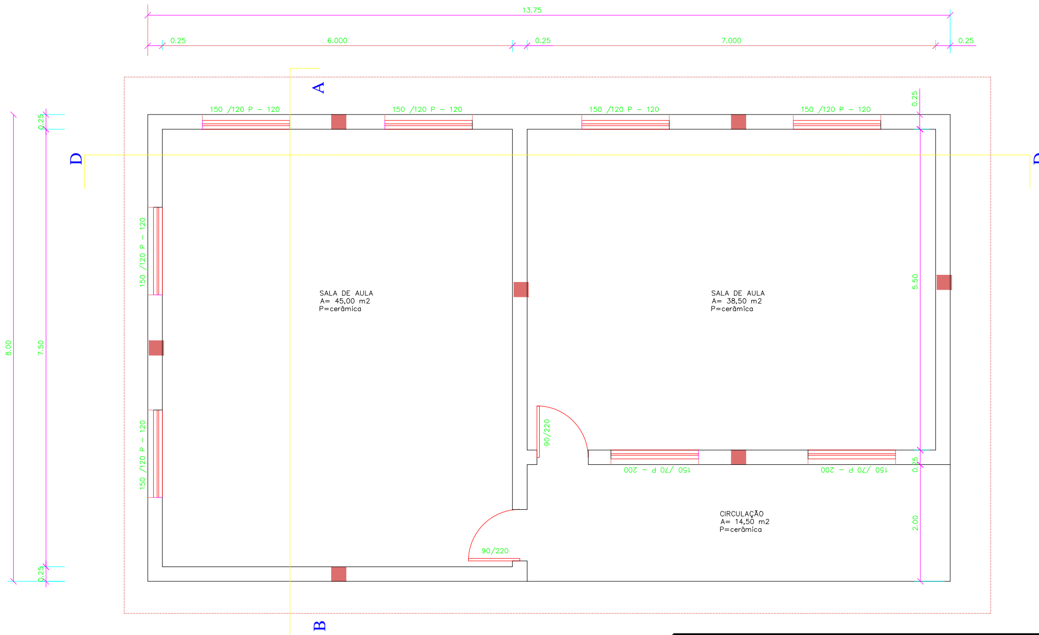
PLANTA BAIXA A: 110,00m 2
