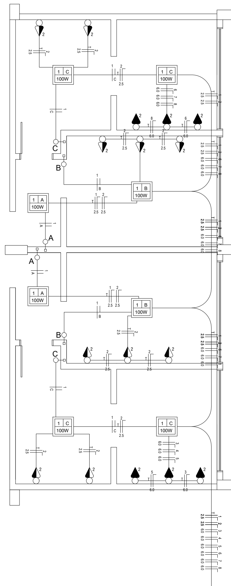
PLANTA ELÉTRICA - DETALHE VESTIÁRIOS RETIFICADA
