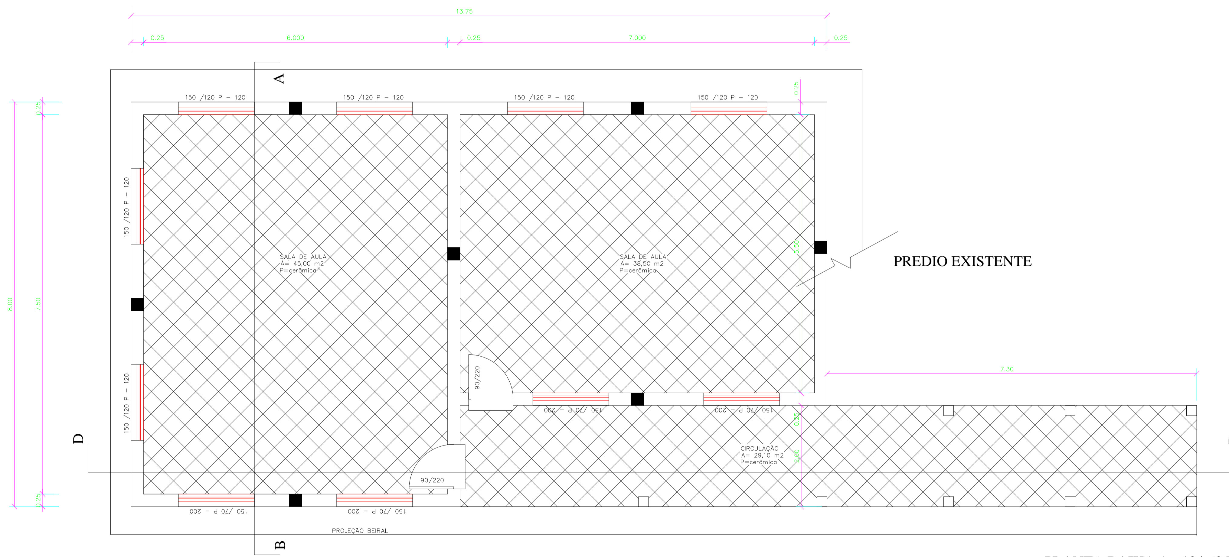
PLANTA BAIXA A= 124,60 M2
