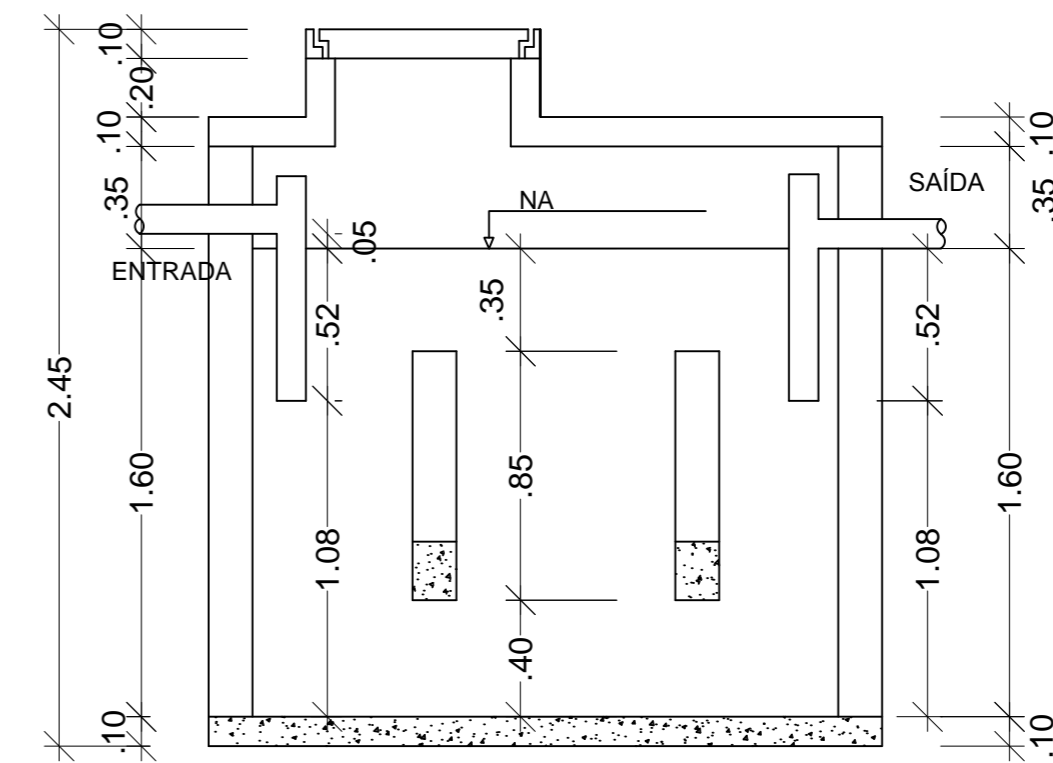
CORTE AA
