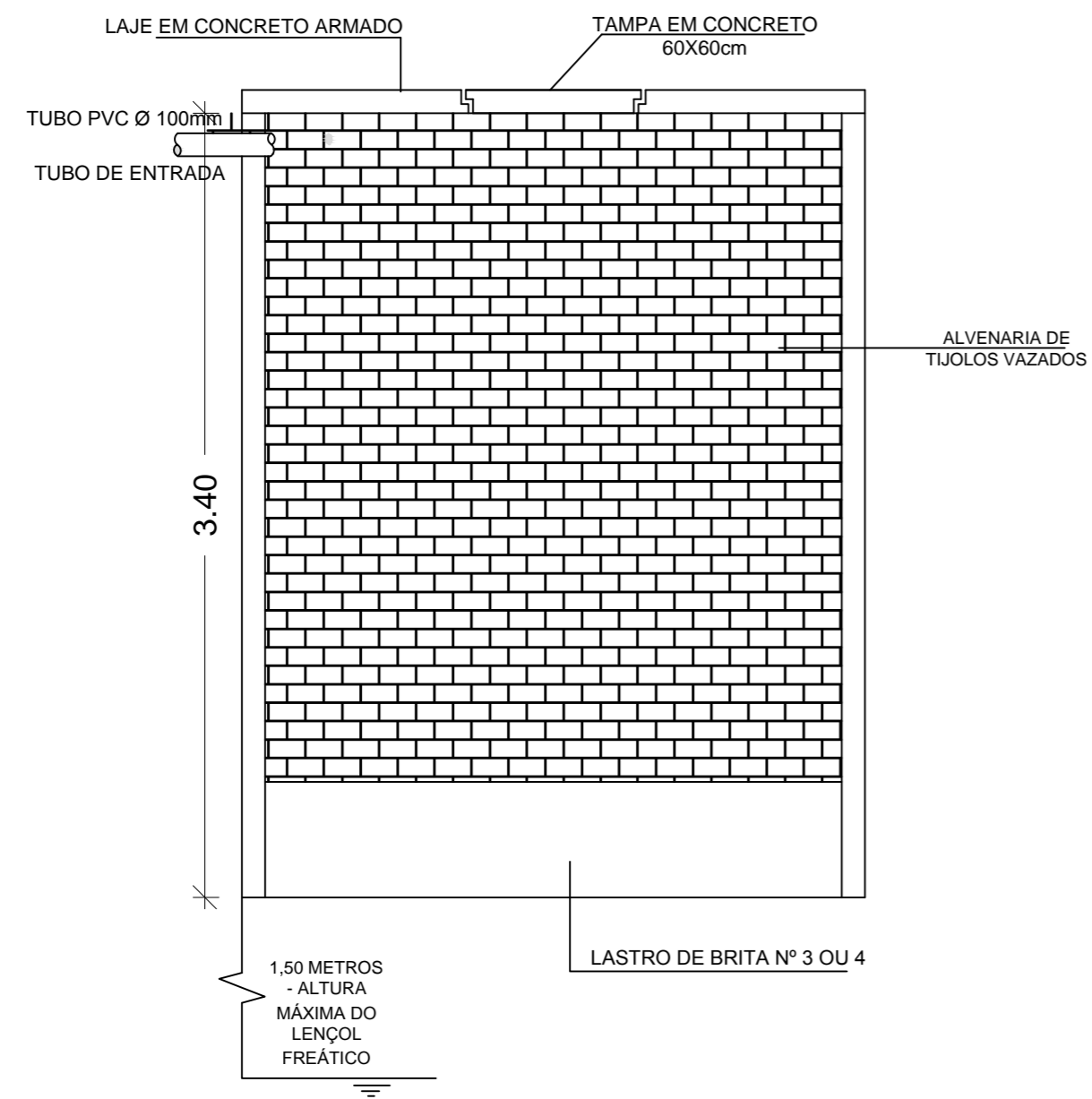
CORTE AA
